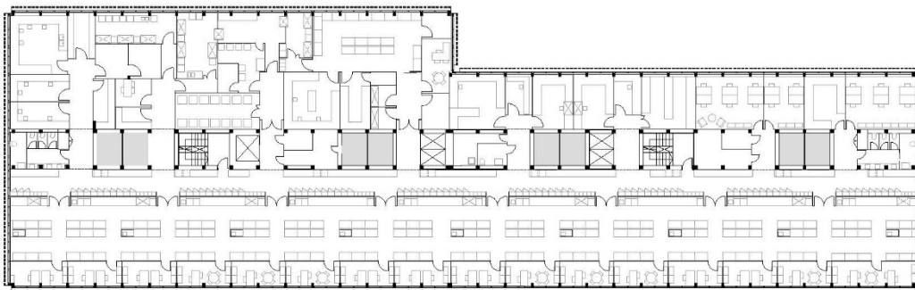
Planta segona. Imatge: PICHarchitects_Pich-Aguilera
